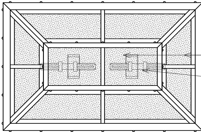
BOTTOM
